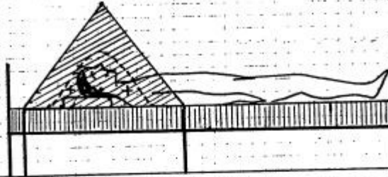
Fig. 2. Position in nach unten reflektierter erster Pyramide im negativen Energiezentrum.
